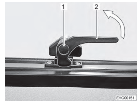
Fig. 40 Palanca de bloqueo inferior (posición "cerrada")
