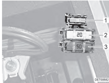
Fig. 105 Fusibles en la batería del motor de arranque sin amplificador de carga
