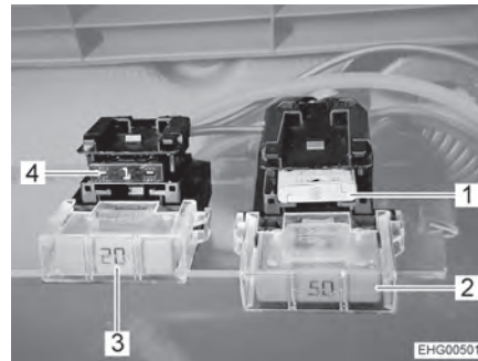
Fig. 108 Fusibles en la batería del habitáculo con amplificador de carga (Fiat/Citroën)
