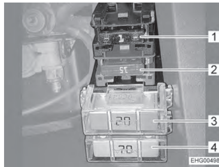
Fig. 106 Fusibles en la batería del motor de arranque con amplificador carga
