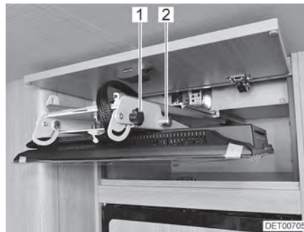
Fig. 66 Pantalla plana en el compartimento de televisor
