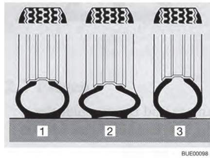
Fig. 172 Superficie de contacto del neumático
