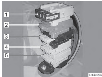
Fig. 112 Fusibles junto al bloque eléctrico con preparación para energía solar e instalación de antena parabólica
