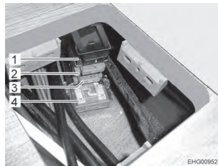
Fig. 109 Fusibles en la batería del habitáculo con amplificador de carga (Ford)
