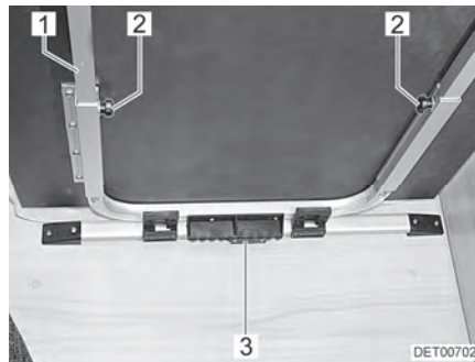
Fig. 58 Desplazamiento/ampliación de la mesa colgante
