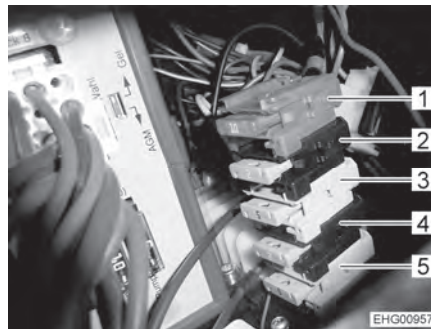
Fig. 111 Fusibles junto al bloque eléctrico (Ford)
