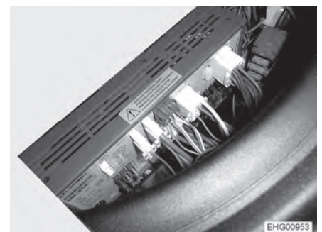
Fig. 99 Lugar de instalación del bloque eléctrico (Ford)
